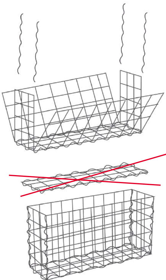
NESPRÁVNA MONTÁŽ
