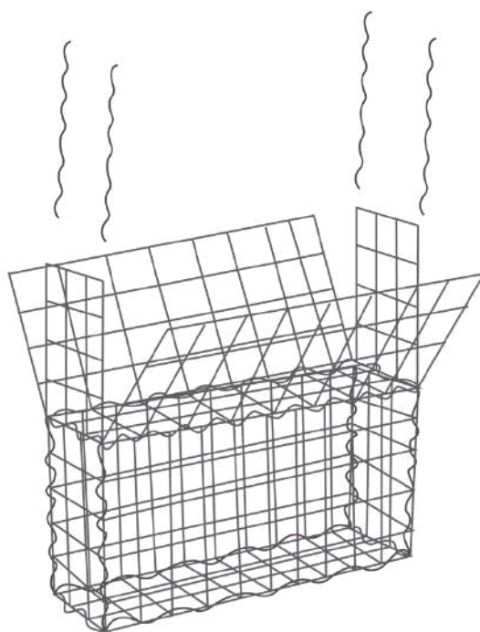
SPRÁVNA MONTÁŽ
